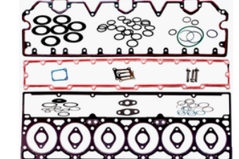
JGO. DE EMPAQUE DE ALTA (CULATA)
