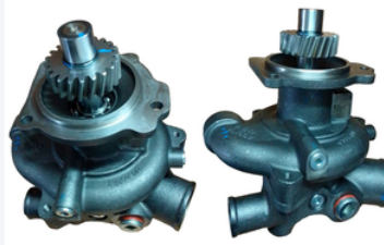
BOMBA DE AGUA - EJE CORTO
